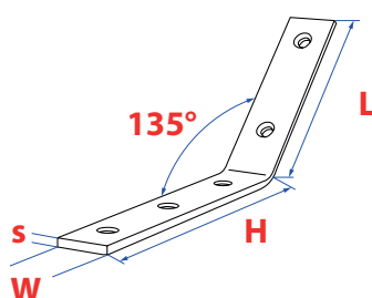
Equerre asymétrique - 135° Winkelverbinder - 135°
