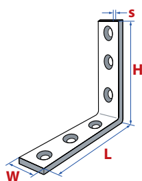
Equerre porte - Type lourde Winkelverbinder schwer
