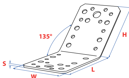
Equerre d'assemblage - 135° Strebenverbinder - 135°
