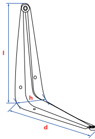
Console emboutie - Type 1 Blechkonsole - Typ 1
