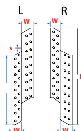
Pattes de solivage - gauche + droite Sparrenpfettenanker - Links + Rechts
