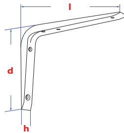
Console emboutie - Type 2 Blechkonsole - Typ 2
