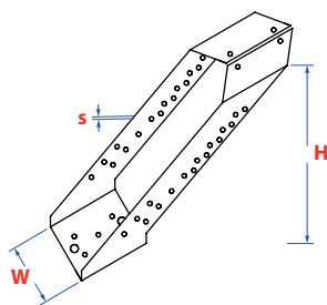
Cantilever Balkenverbinder
