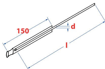
Tige de dilatation lisse Gleitanker
